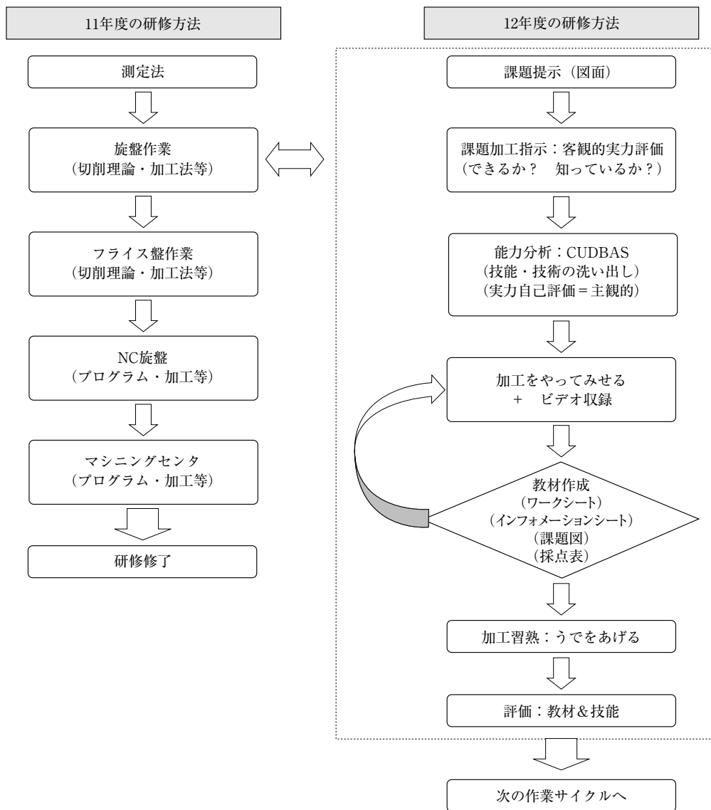
図5 研修の流れ
