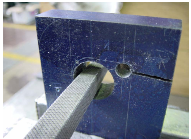
Cクランプヤスリ作業
