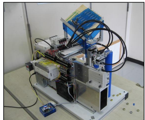
(e) 試作機外観
