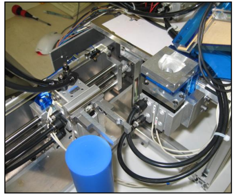
(f) 組立・搬送部周辺
